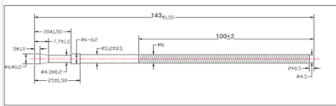
Wedge Anchor Fastner M6
